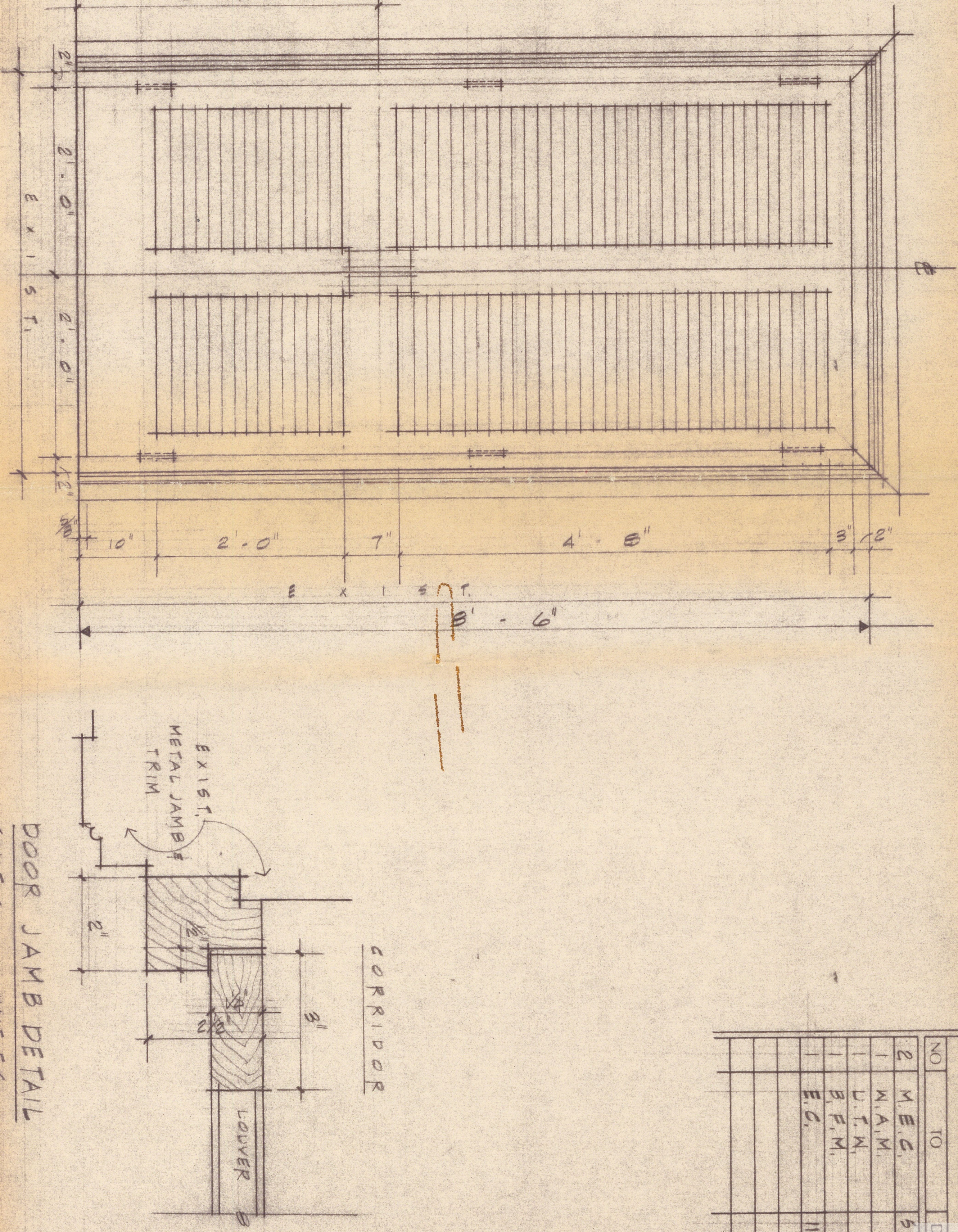
DOOR ELEVATION SCALE: 1/2" = 1'-0"
